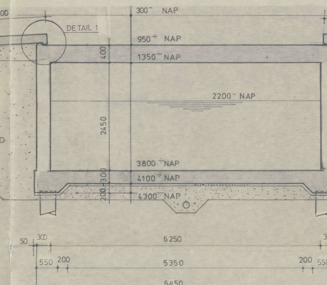
DOORSNEDE B-B
