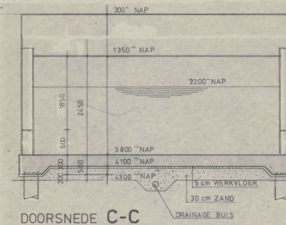
DOORSNEDE C-C
