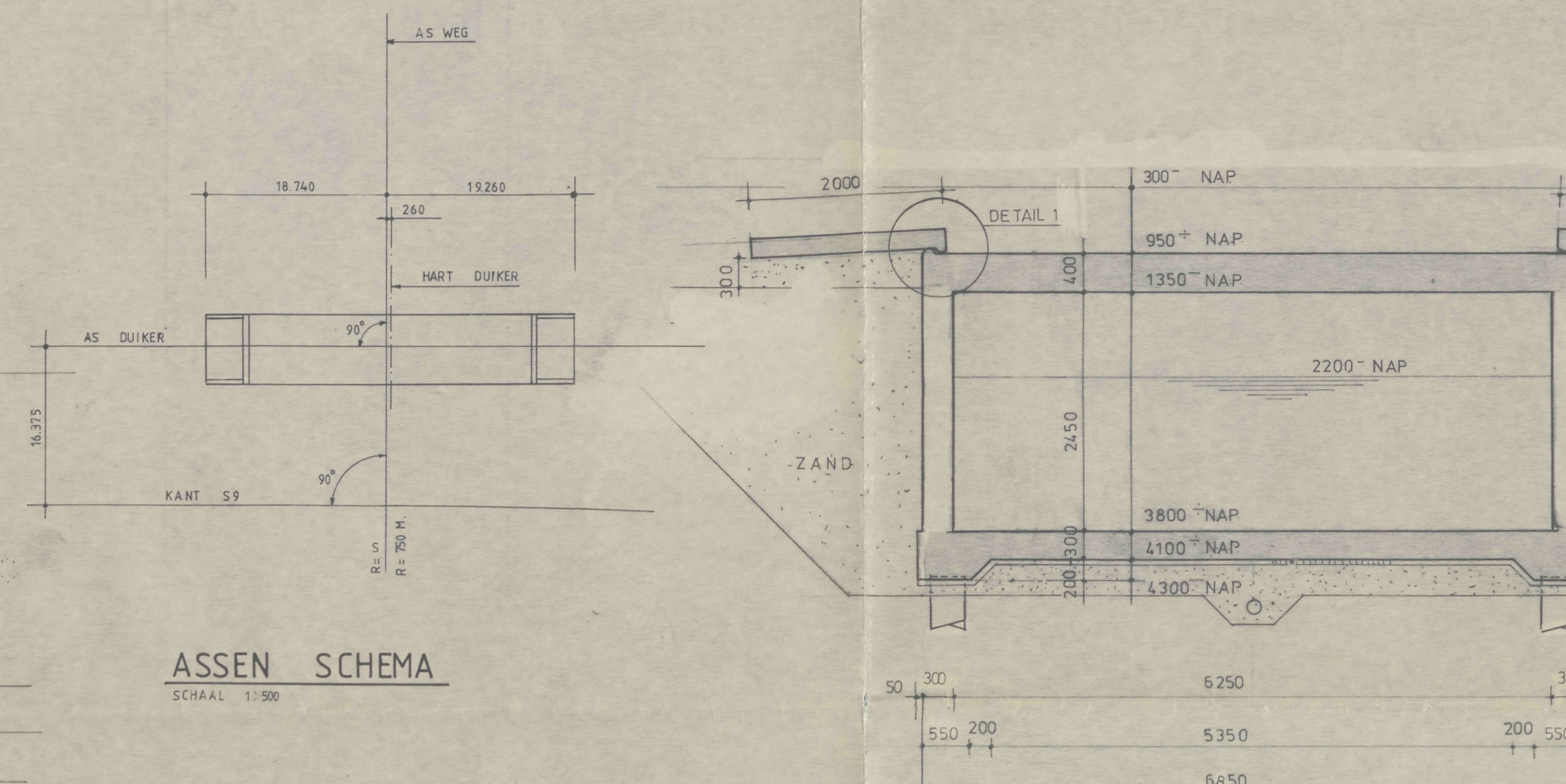
DOORSNEDE B-B
