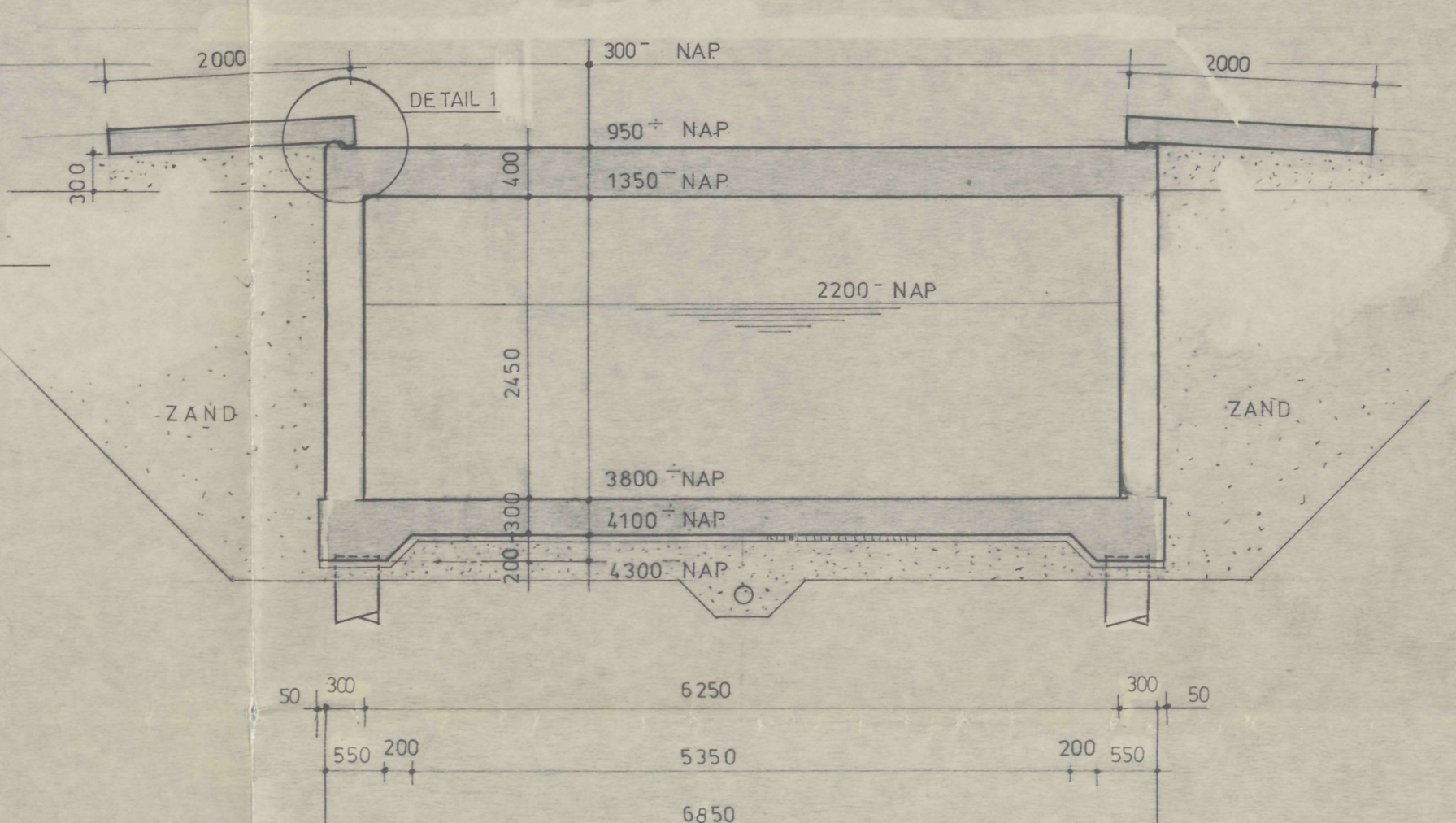
DOORSNEDE B-B
